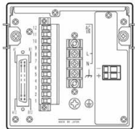
背面(矢視A)
