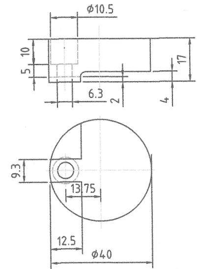
金具 B1C
