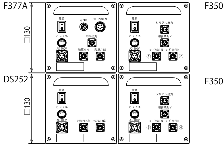
背面 (矢視 A)
